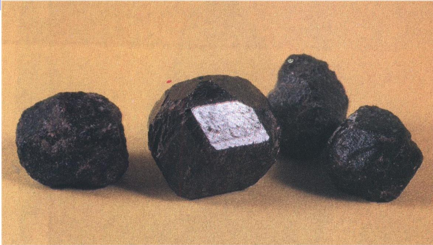
Альмандин(4 кристали). Україна.
