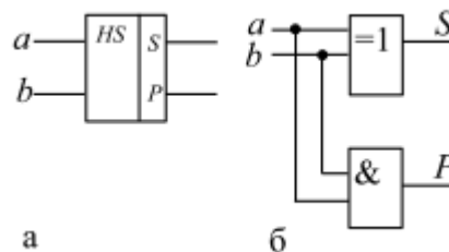
Рис. 7.1. Графічне позначення (а) та схема (б) напівсуматора.
