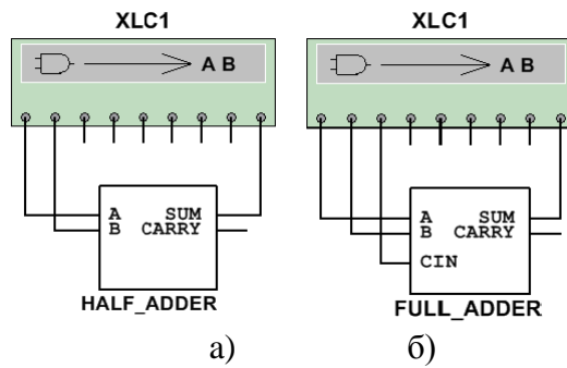
Рис. 7.6. Приклад під'єднання напівсуматора (а) та повного суматора (б) до логічного перетворювача.
