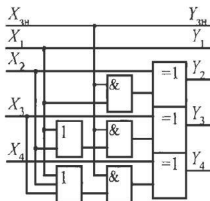
Рис. 7.6. Схема перетворювача прямого коду в доповнювальний.
