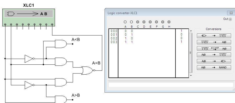
Рис. 7.5. Моделювання схеми однорозрядного цифрового компаратора.
