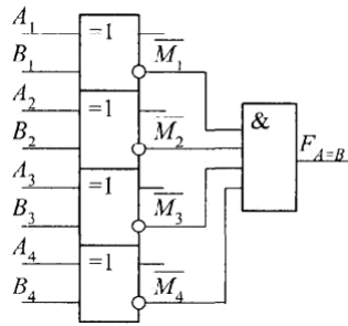
Рис. 7.4. Схема порівняння двох чотирирозрядних чисел A і B .
