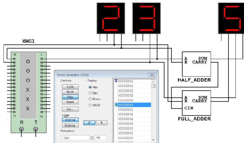
Рис. 7.7. Моделювання дворозрядного суматора.
