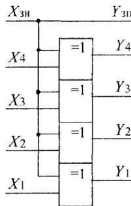
Рис. 7.5. Схема перетворювача прямого коду в обернений.
