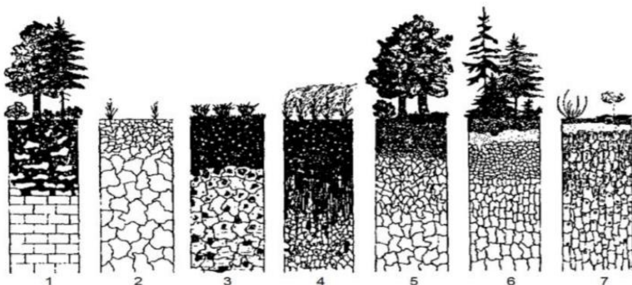
Рис. 3. Головні генетичні типи будови ґрунтового профілю (за Б. Г. Розановим), 2004) Умовні позначення: 1 – гумусовий недиференційований; 2 – безгумусовий; 3 – гумусово-глеєвий; 4 – гумусово-карбонатний; 5 – буроземний; 6 – підзолистий; 7 – солонцевий
