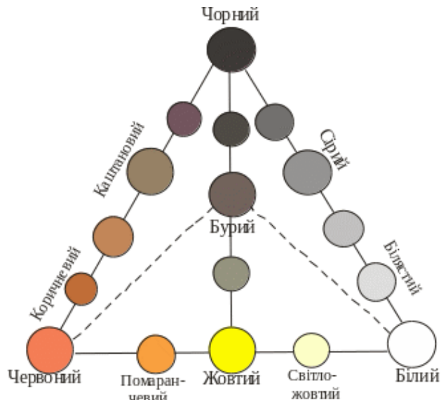
Рис.6. Типи забарвлення ґрунтів (трикутник С.О. Захарова)
