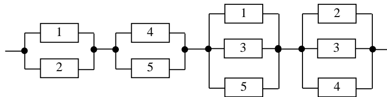
Рис 5.8. Набір мінімальних перетинів
