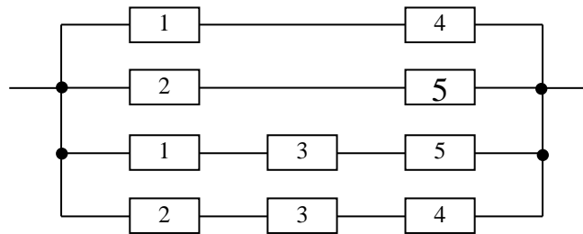
Рис. 5.7. Набір мінімальних шляхів
