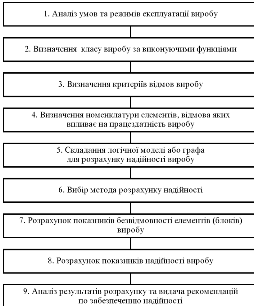
Рис. 6.1. Наближений алгоритм розрахунку надійності при проектування виробу
