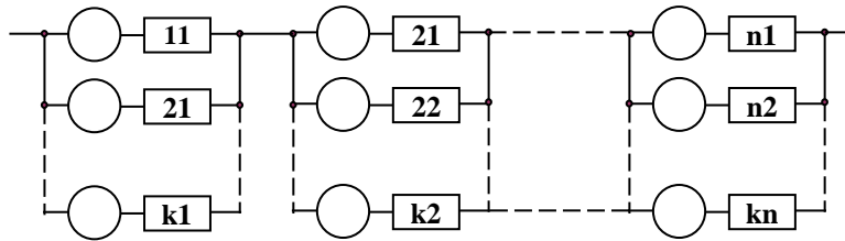
Рис.4.1. Логічна схема системи з активним резервуванням: 1, 2, \dots, n - основні та резервні елементи; \Pi - перемикачі, n - кількість ділянок резервування; k - кількість резервних елементів.
