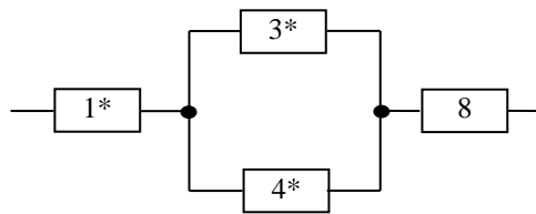
Рис. 5.4. Вигляд схеми після другого перетворення
