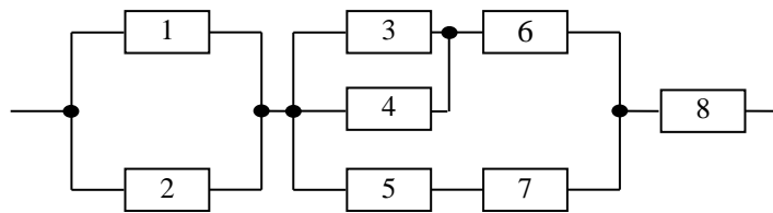
Рис. 5.2. Паралельно-послідовне з'єднання елементів
