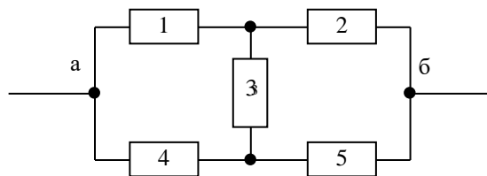
Рис. 5.11. Логічна схема складної системи для розрахунку надійності
