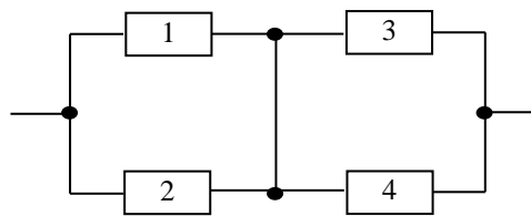
Рис 5.1. Паралельно-последовне з'єднання елементів
