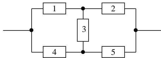
Рис. 5.6. Мостова схема
