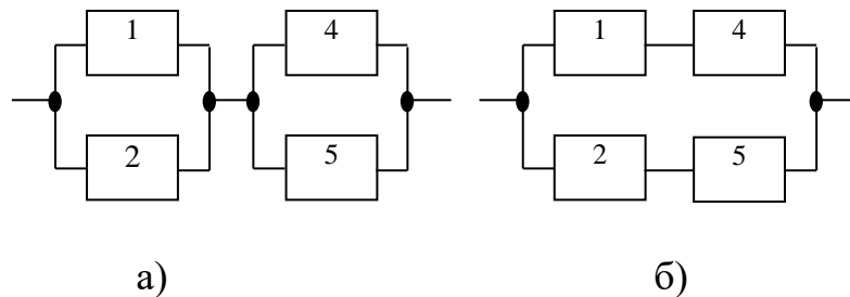
Рис 5.9. Вид мостової схеми після перетворення: а) паралельно-послідовне з'єднання елементів ( x_3 = 1 ); б) послідовно-паралельне з'єднання елементів ( x_3 = 0 ).
