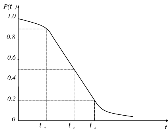
Рис. 2.1. Визначення гамма-відсоткового строку збережності
