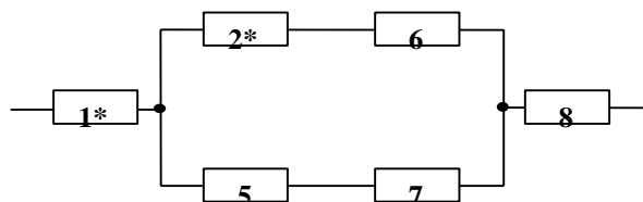
Рис. 5.3. Вигляд схеми після першого перетворювання формулами
