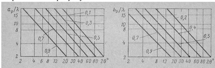
Рисунок 6.2 – Залежність розмірів розкриву оптимального рупора від потрібної ширини ДН при різних відносних рівнях (за напруженістю поля)
