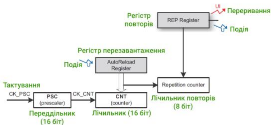
Рис. 3.4. Частина блок-діаграми таймера загального призначення
