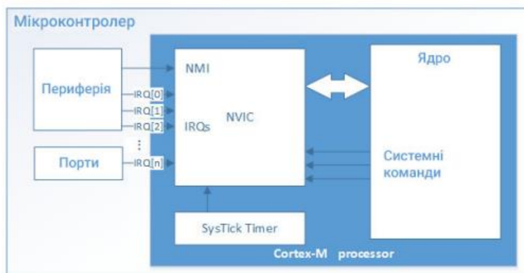
Рис. 3.3. Схема обробки переривань в мікропроцесорах Cortex
