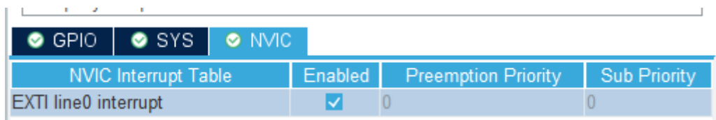
Рис. 3.9. Встановлення дозволу на зовнішні переривання
