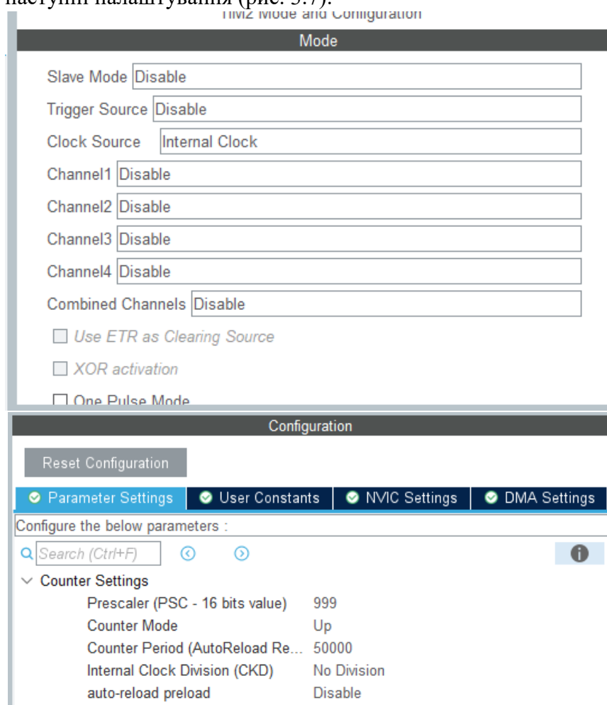
Рис. 3.7. Налаштування таймера для генерування переривання з періодом 0,5 с
