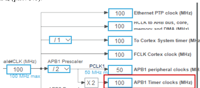
Рис. 3.6. Частоти тактування на шинах APB1 та APB2
