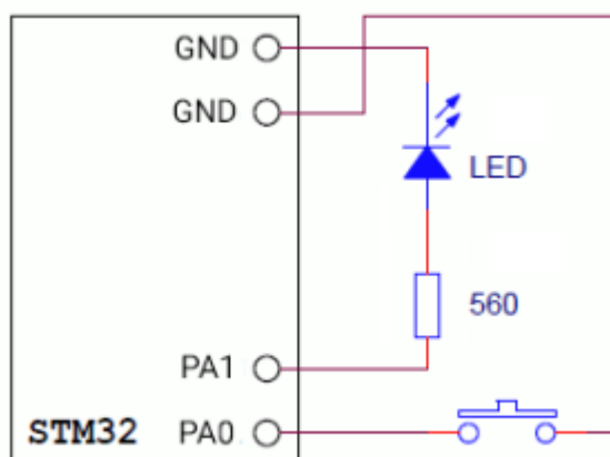
Рис. 3.5. Підключення зовнішнього світлодіода та кнопки
