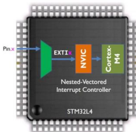
Рис. 3.2. Зовнішнє переривання на виводі мікроконтролера
