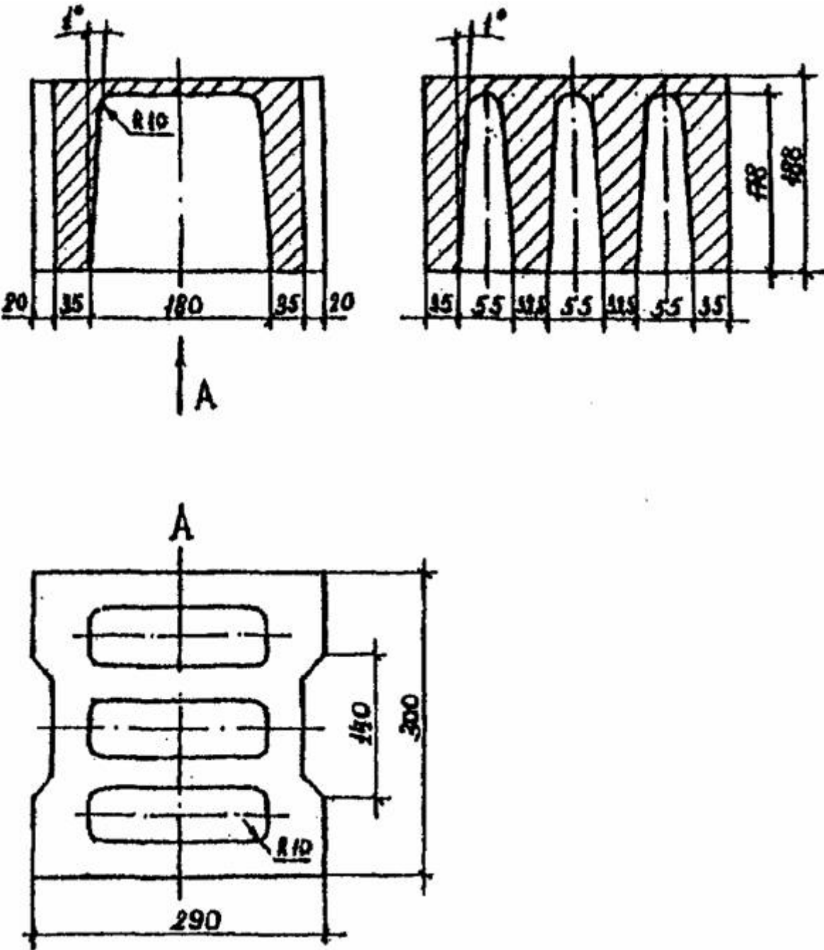
Рисунок Б.5 - Блок порожнистий із горизонтальною діафрагмою
