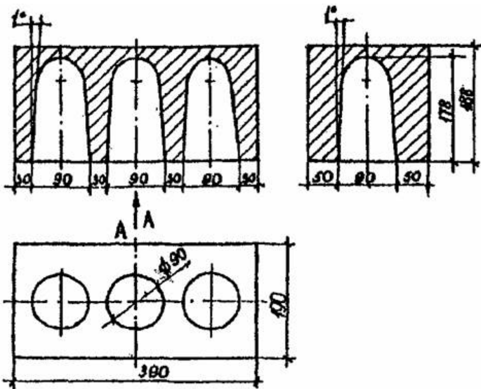
Рисунок Б.3 – Блок порожнистий із горизонтальною діафрагмою
