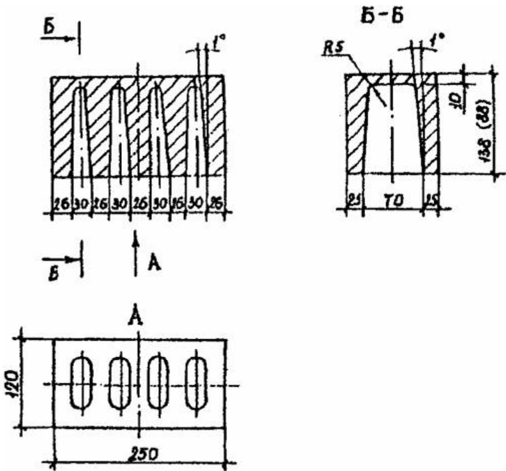
Рисунок А.3 - Камінь порожнистий із горизонтальною діафрагмою
