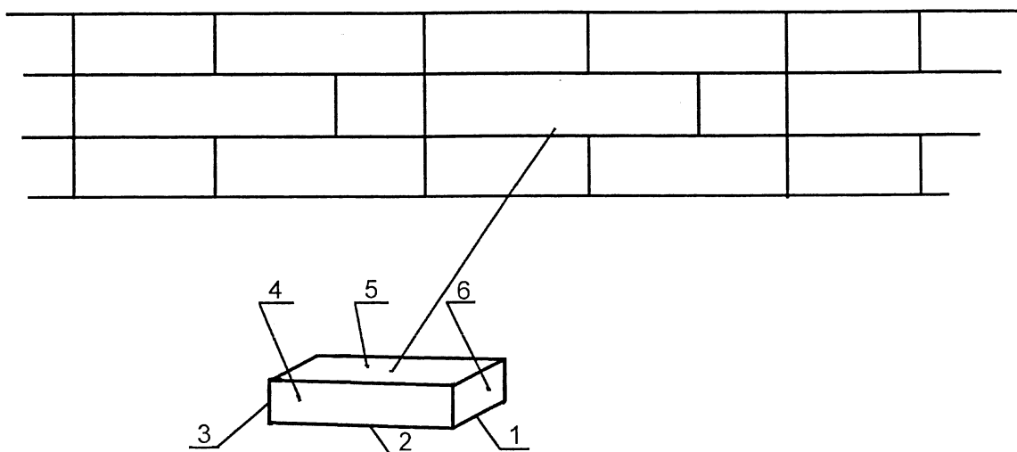
Рисунок 1 – Фрагмент стіни
