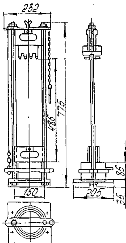
Рисунок 7 - Копер ПМ
