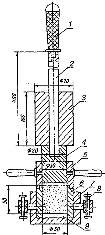
1 - рукоятка; 2 - направляющий стержень; 3 - гиря; 4 - плунжер; 5 - направляющий насадный цилиндр; 6 - разъемный цилиндр; 7 - подстанник; 8 - закрепляющие винты; 9 - металлическая пластинка
