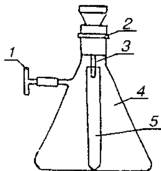
Рисунок 11 - Устройство для сбора фильтрата
