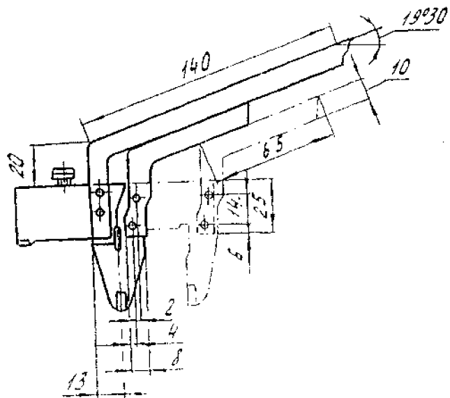
Рисунок 3 - Передвижной шаблон
