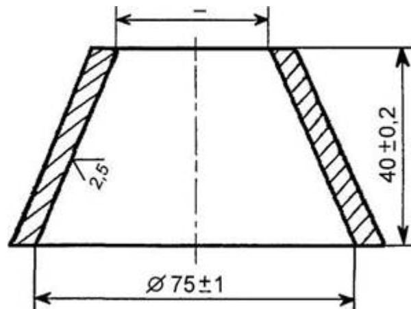
Рисунок 4 - Кільце до приладу Віка
