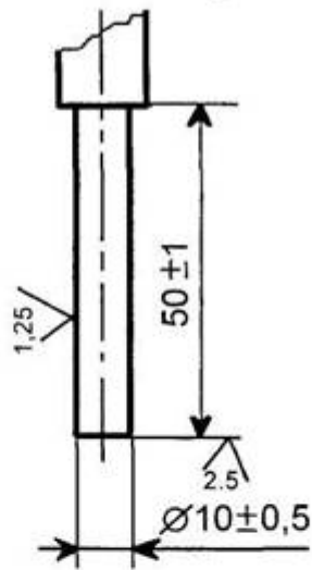
Рисунок 2 – Робоча частина товкачика
