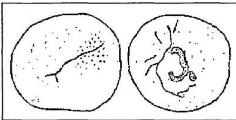
Рисунок 6 - Коржики, що витримали випробування на рівномірність зміни об'єму
