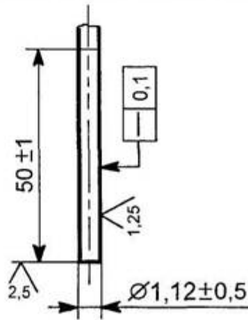
Рисунок 3 - Робоча частина голки
