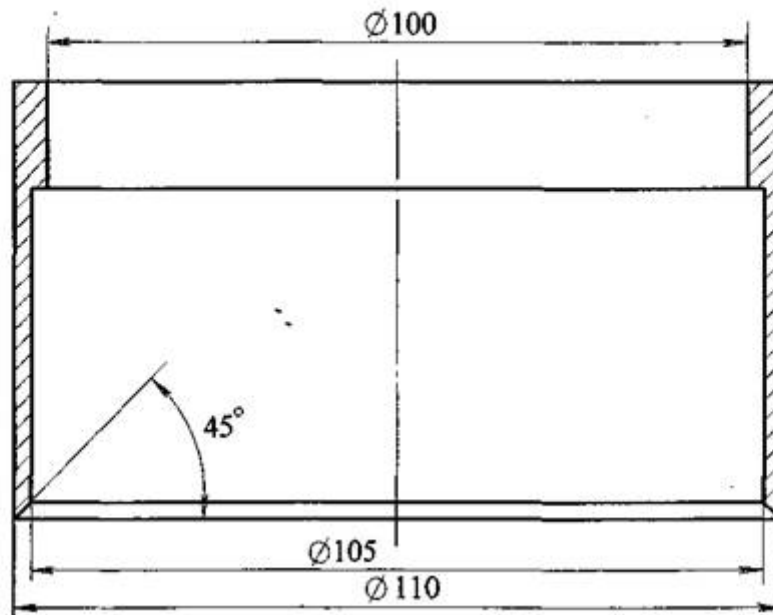
Рисунок В.1 - Металева циліндрична обойма
