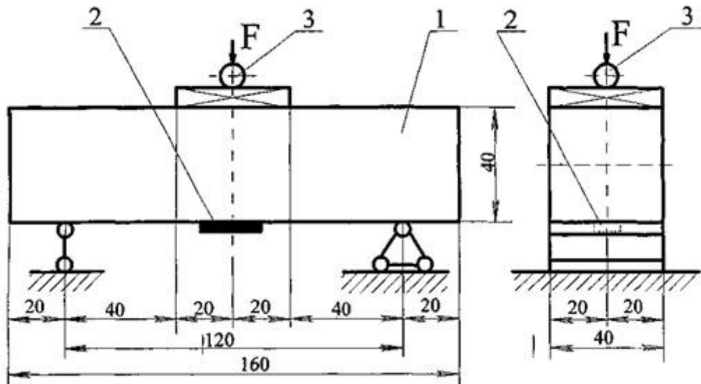
1 - зразок бетону; 2 - тензорезистор; 3 - електричний силовимірювач
