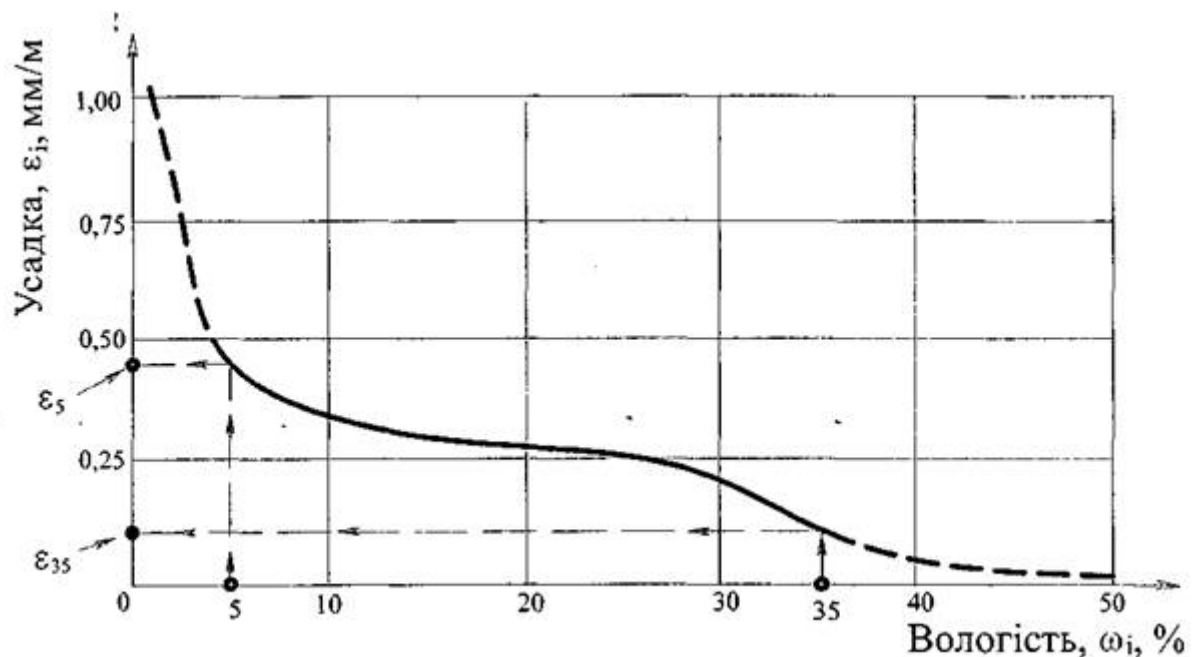
Рисунок А.3 - Приклад графіка усадки бетону
