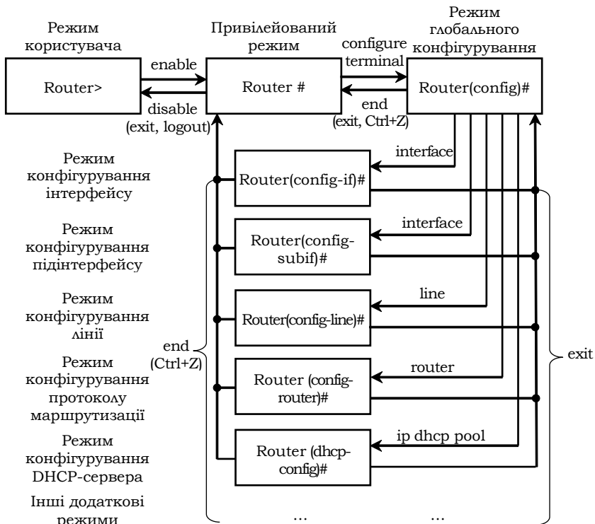
Рис. 10. Командні режими маршрутизатора Cisco та команди переходів між режимами
