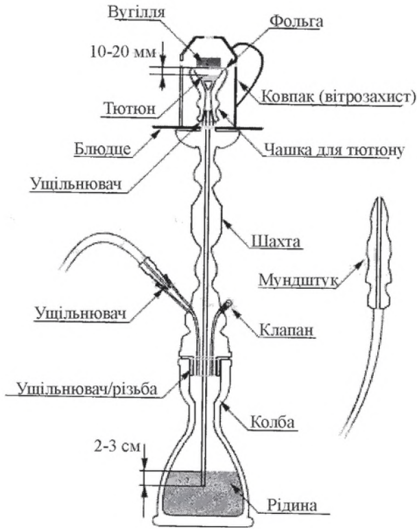
Рис. 2.42. Будова кальяну
