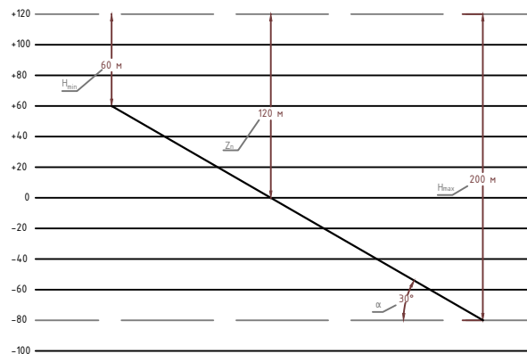
Визначення меж охоронного цілика на вертикальному розрізі вхрест простягання
