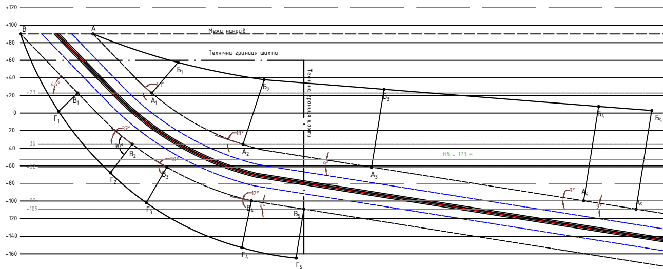
Побудова запобіжного цілика для захисту залізниці способом перпендикулярів
