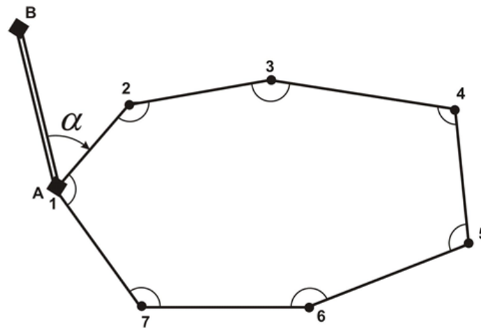
Рис 2. Схема стандартного замкнутого ходу
