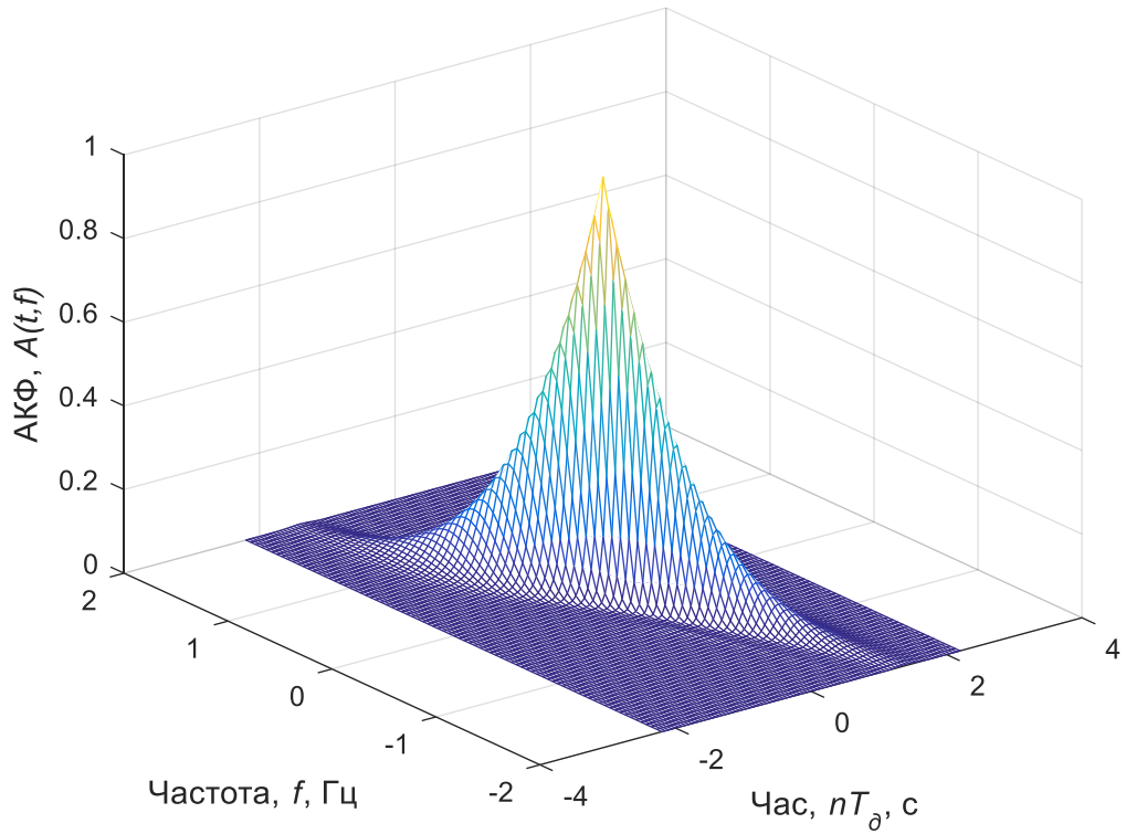
Функція невизначеності для ЛЧМ-імпульсу
