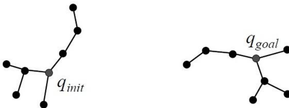
Рис. 11.13. Одична ітерація алгоритму RRT-Connect
