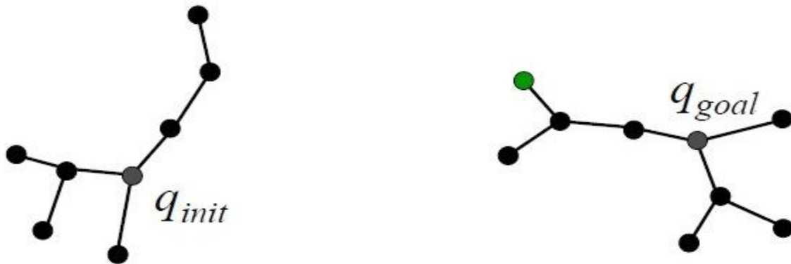
Рис. 11.14. Довільне розширення одного із дерев
