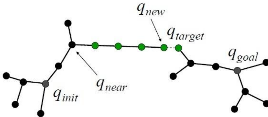
Рис.11.19. Продовження розширення вітки
