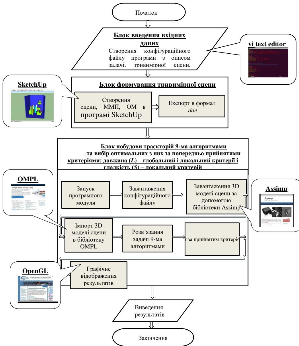
Рис. 11.24. Структурна схема функціонування розробленого ПП “LSTr”
