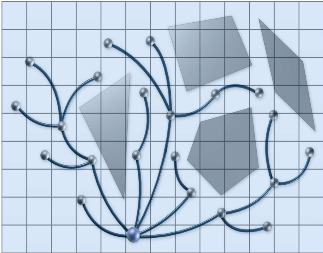
Рис.11.1. Спроцен схема роботи алгоритму A1 - KPIECE
