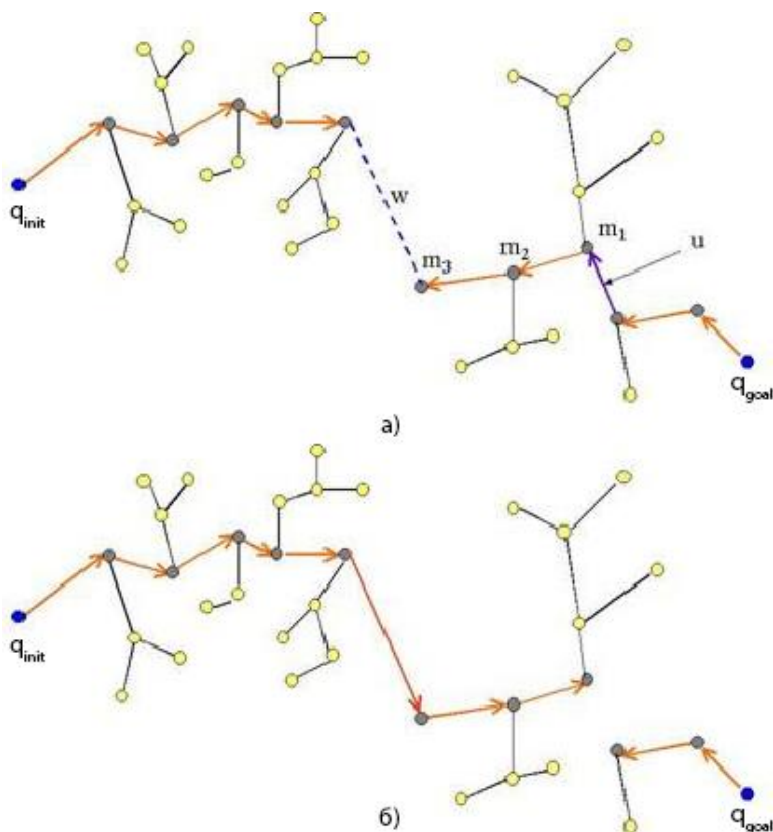
Рис.11.8. Процес перенесення точок з одного дерева в інше в алгоритмі SBL
