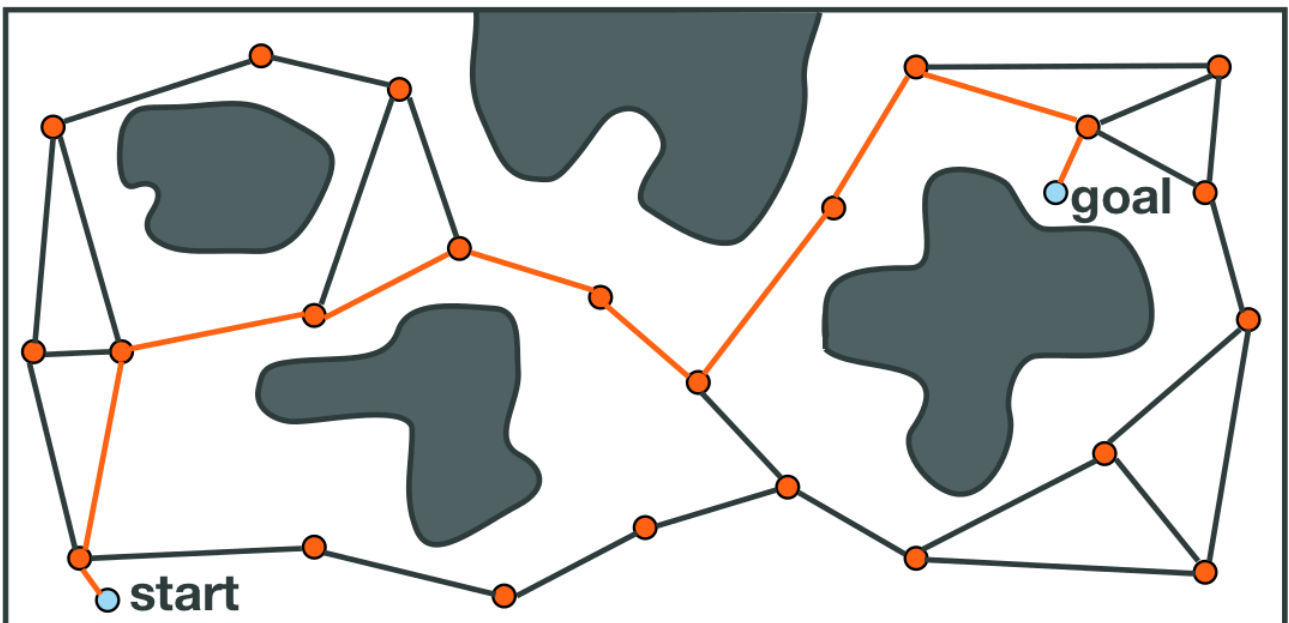
Рис.11.7. Приклад побудови траєкторії PRM алгоритмом. Початкова і кінцева точка з'єднані та найкоротший шлях в графі знайдений
