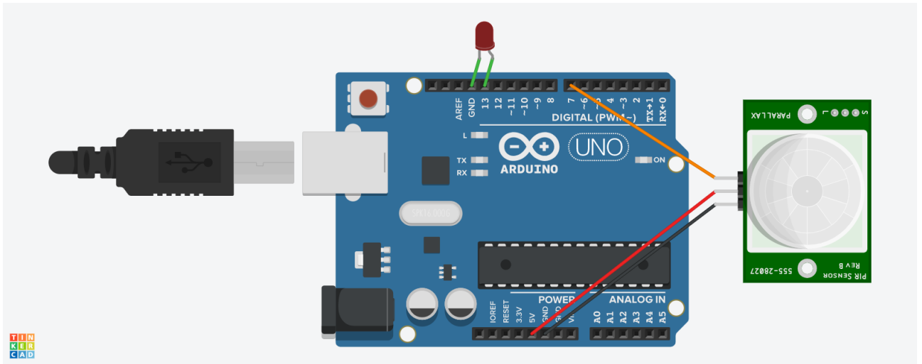
Рисунок 9.3– Схема підключення датчика присутності та світлодіода до Arduino UNO
