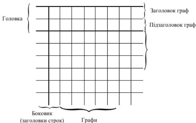
Рис. 3.1. Структура таблиці
