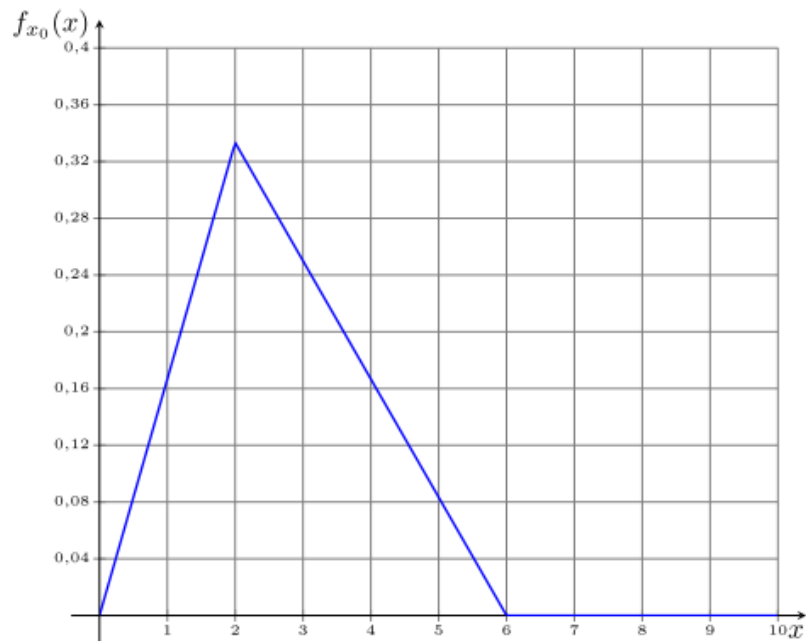
Рис. 11. Приклад графіка функції щільності трикутного розподілу випадкової величини ( a = 0 , c = 2 , b = 6 )
