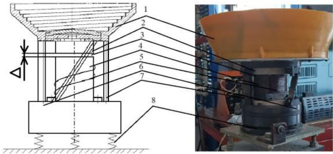
Рис. 1.1. Складові ВБЗП:
