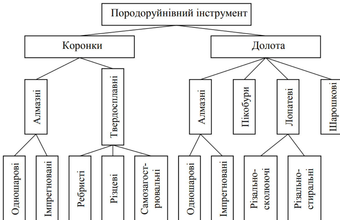
Рис. 1 – Схема класифікації породоруйнівного інструменту
