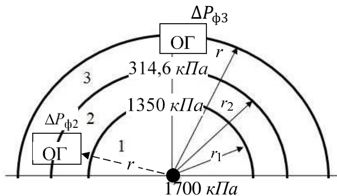
Рис. 3.1. Зонування територій під час вибуху ГПС
