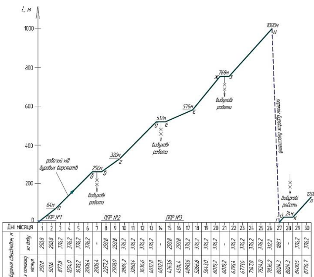
Рис. 5. Графік організації роботи бурового верстата
