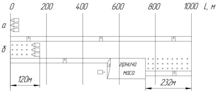
Рис. 4. Розташування бурових верстатів на уступі: а – на початок місяця; б – на кінець місяця
