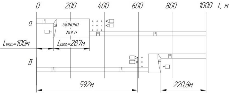
Рис. 6. Розташування мехлопати і бурових верстатів на уступі:
