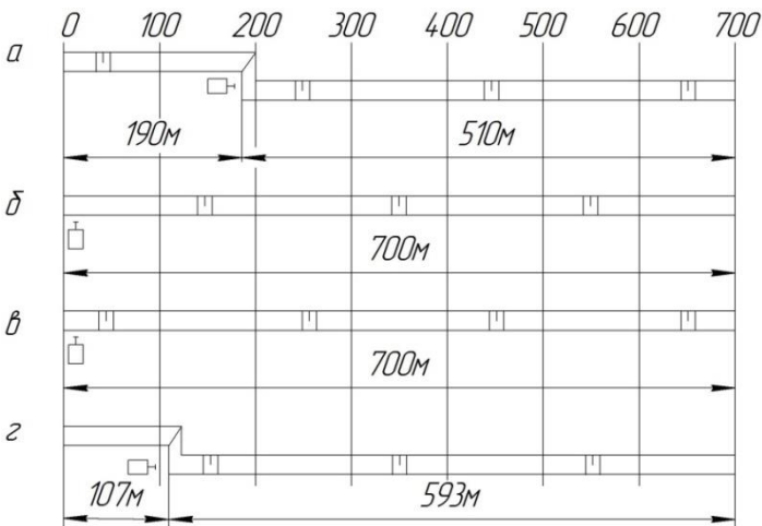
Рис. 2. Ескізи розташування екскаваторного вибою
