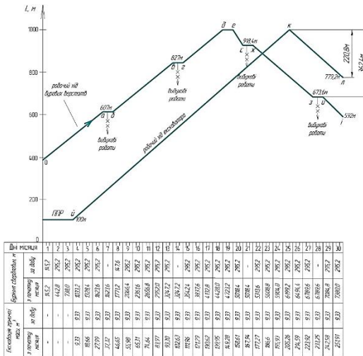
Рис. 7. Графік організації роботи бурових верстатів і мехлопати
