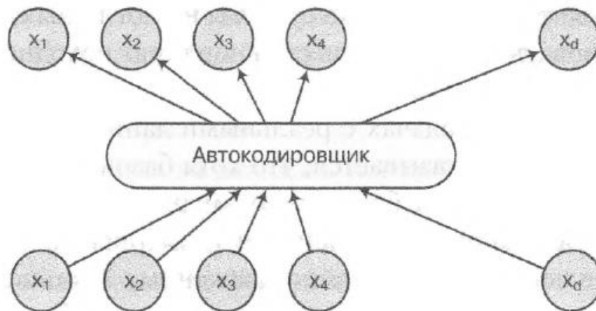
Рис.3. Як працює автокодувальник
