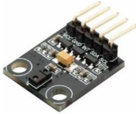
Рис. 3.2. – Зовнішній вигляд датчика кольору RobotDun APDS-9960
