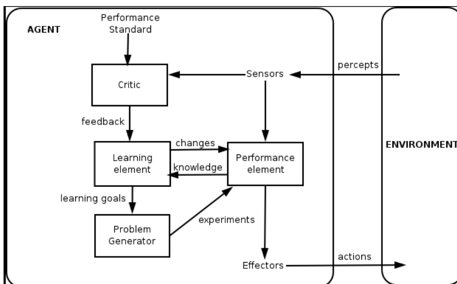
Рис. 2. Інтелектуальний агент
