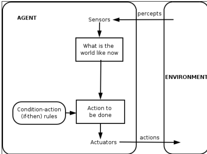
Рис. 1. Звичайний агент
