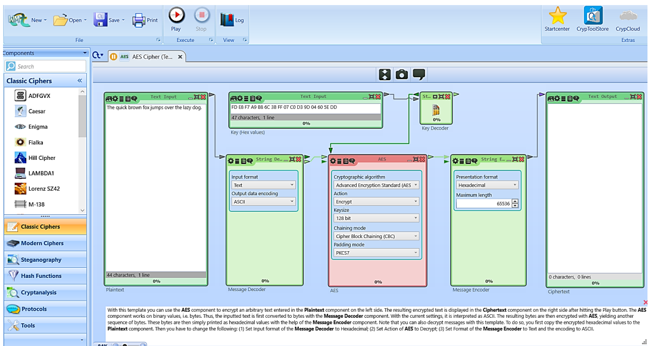
Рис. 4.1. Шаблон проекту, що реалізує шифрування тексту за алгоритмом AES
