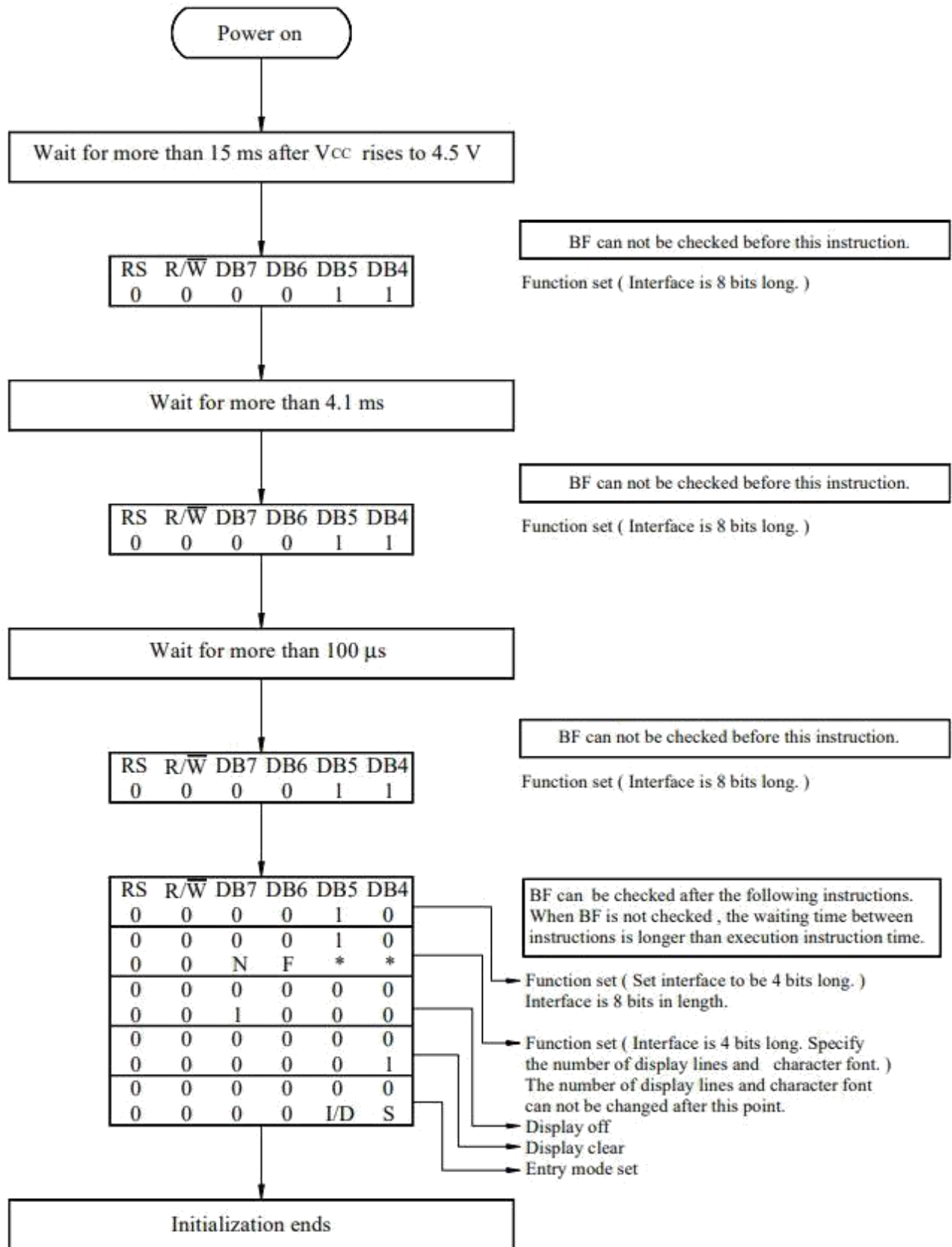
Рис. 3.16. Блок-схема процесу ініціалізації символного екрану в чотирьохрозрядному режимі передачі даних
