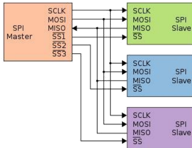
Рис. 3.10. Схема включення «один ведучий – кілька незалежних підлеглих»
