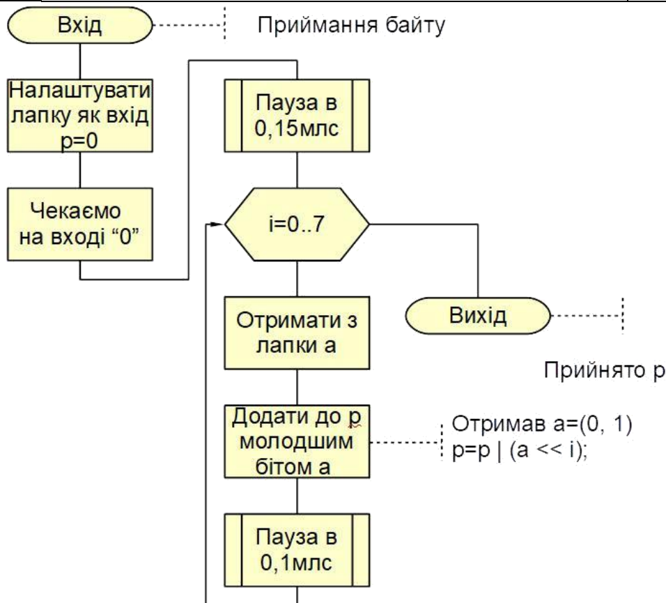
Рис. 3.8. Алгоритм прийому байту з послідовного USART порту
