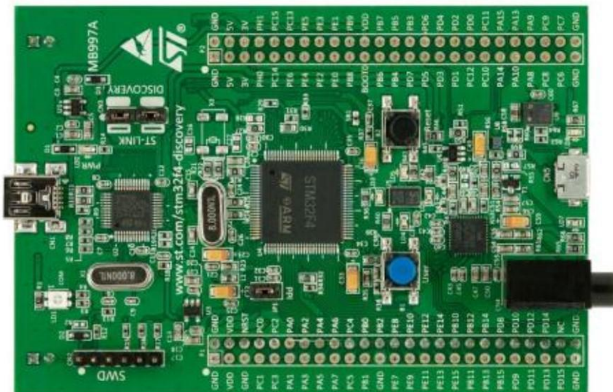
Рис. 1.3. Зовнішній вигляд плати STM32F4Discovery
