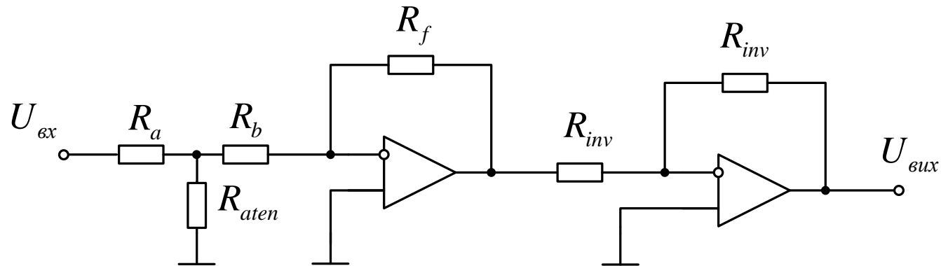
Неінвертуючий атенюатор без зміщення нуля
