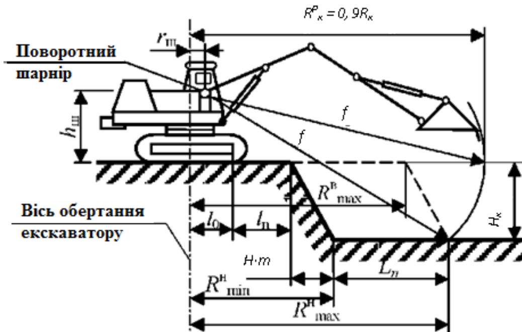
Рис. 2.7. Визначення параметрів екскаватора
