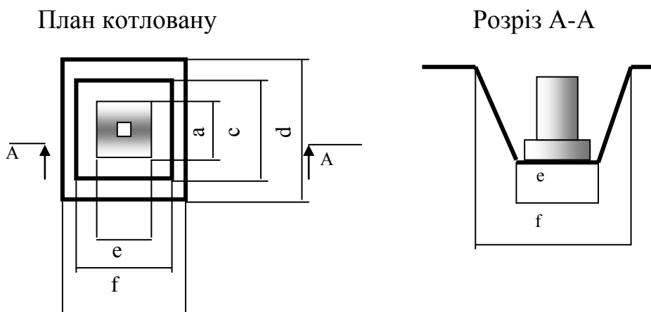
Рис. 2.2. Розміри котловану.
