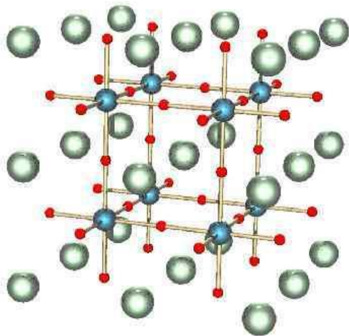
Структура YAlO_3
