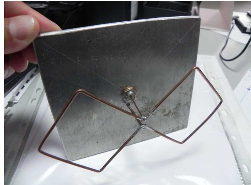
Антенa Харченко з рефлектором
