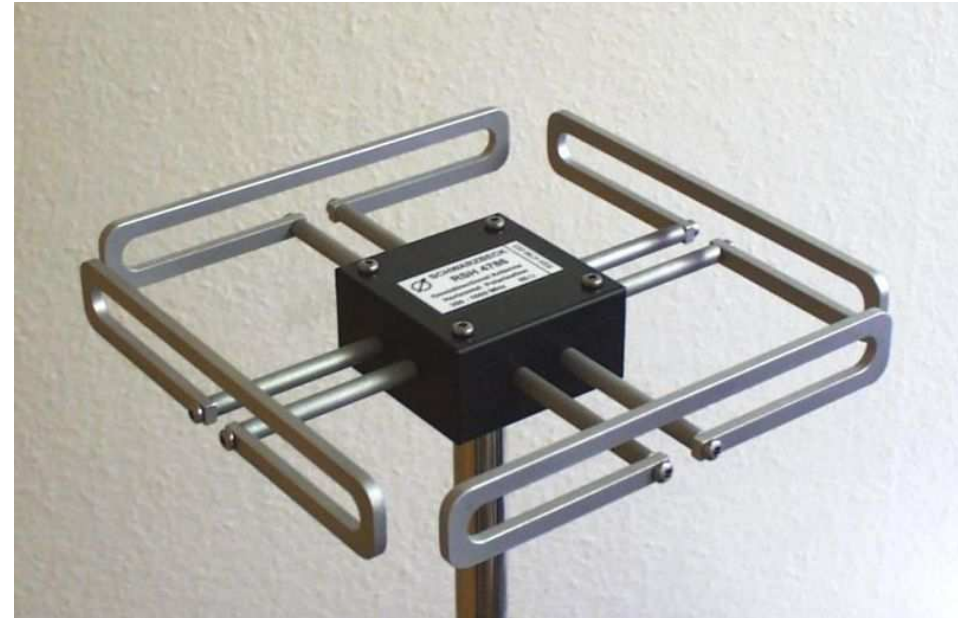
Горизонтальна всепрямована антена, модель RSH4786 (фірма Schwarzbeck)
