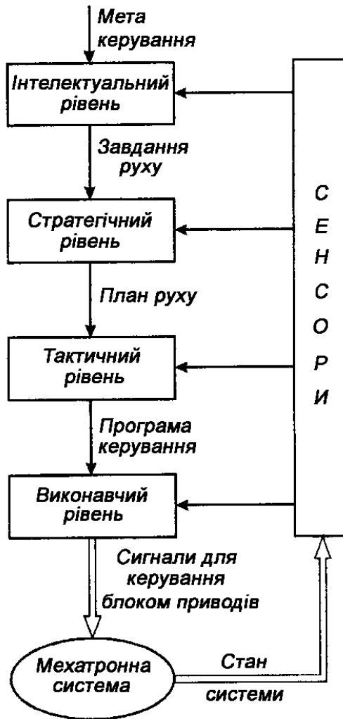
Рис. 7.1 – Рівні керування в МТС та ПР
