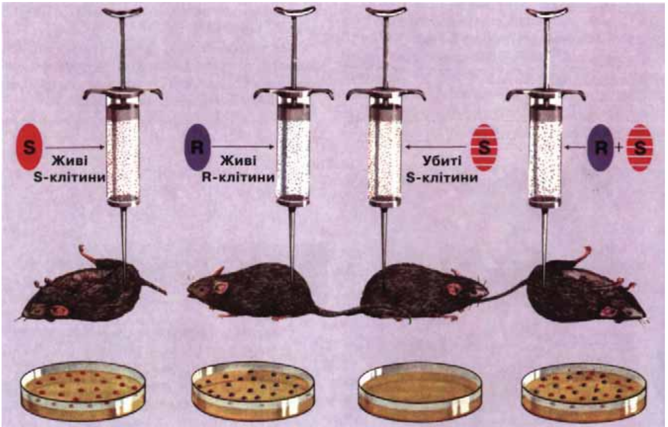
Рис. 1.47 Трансформація.
