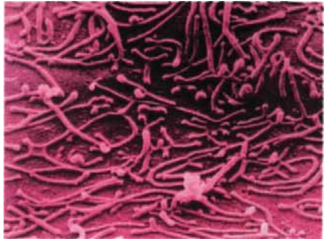
Рис. 1.5 Мікоплазма (мікрофотографія).
