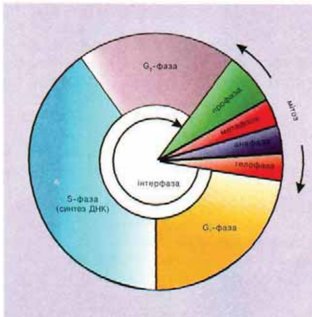
Рис. 1.73 Клітинний цикл.
