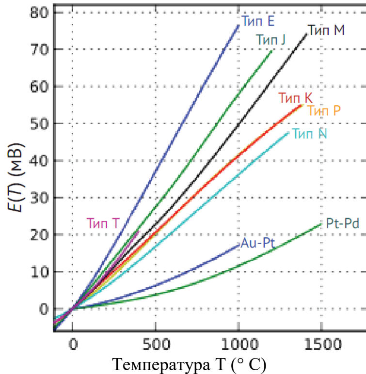
Рис. 3.2. Залежність ЕРС термопар від її температури E(T) : T
