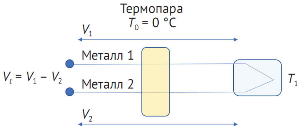
Рис. 3.1. Блок-схема вимірювання температури за допомогою термопари
