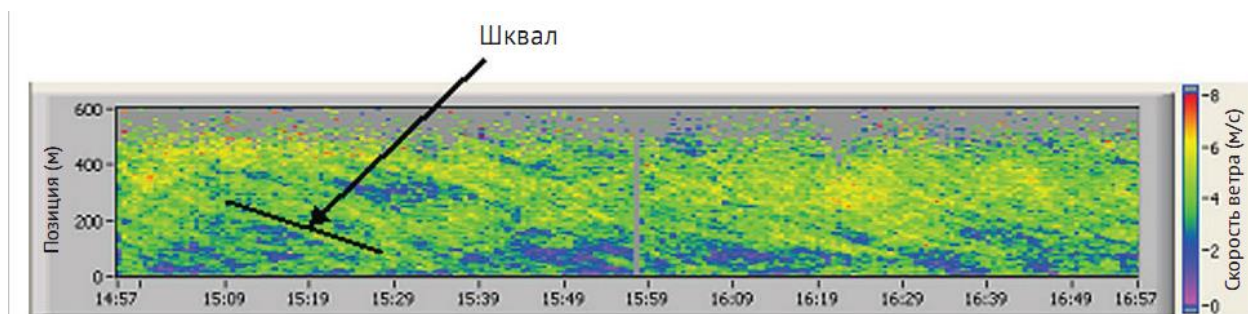
Рис. 3.7 LiDAR: приклад зображення, отриманого за допомогою LiDAR.
