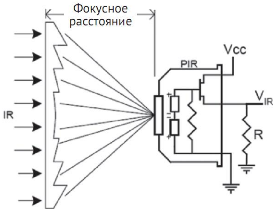
Рис. 3.6 Зліва: лінза Френеля фокусує ІЧ-випромінювання на ПІР-датчик. Схема по застосуванню Cypress Microsystems AN2105
