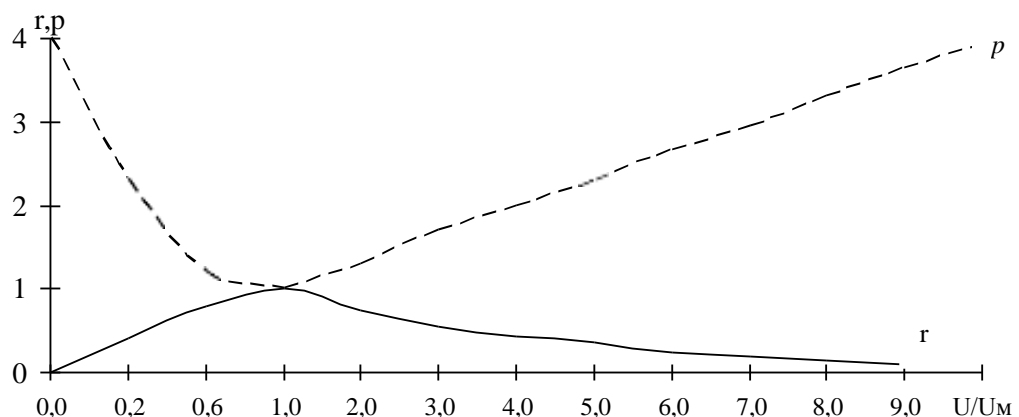
Рис.2.3 Графік для визначення безрозмірного коефіцієнта r і p в залежності від швидкості вітру.
