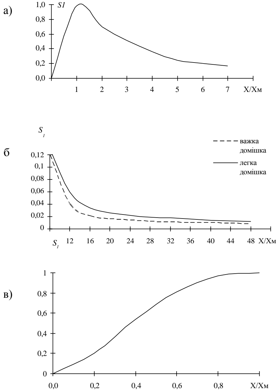
Рис.2.1 Графік визначення безрозмірного коефіцієнта S_I
