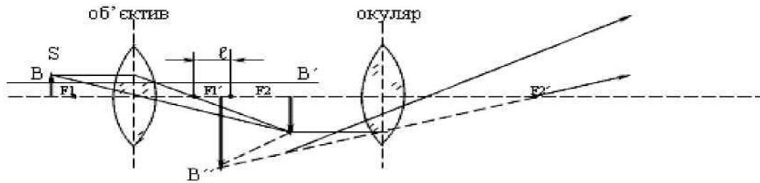
Рис. 2.4. Хід променів у світловому мікроскопі.
