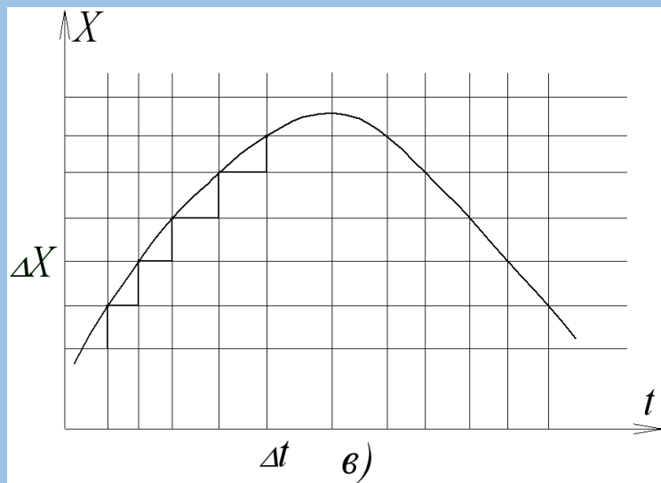
Рис.1. Види квантування сигналу: a – за рівнем, б – за часом, в – за часом та рівнем.
