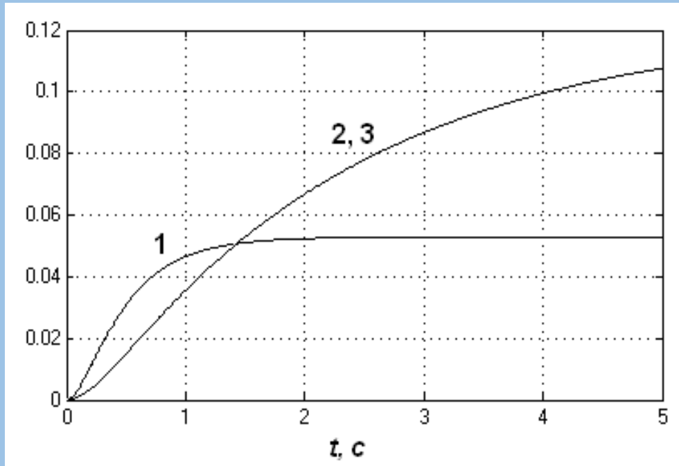
Рис.10. Перехідні та імпульсні характеристики цифрових САУ, перетворених різними методами: 1- метод c2d , 2,3- методи bilinear та impinvar
