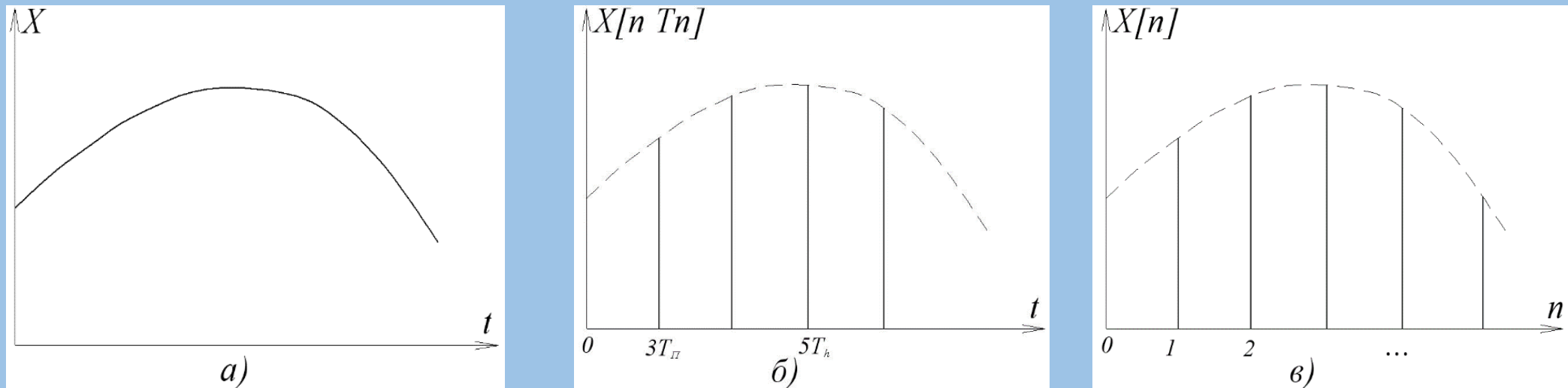
Рис.4. Решітчасті функції: а – неперервний сигнал; б, в – форми представлення решітчастих функцій
