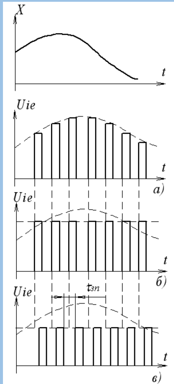
Рис.3. Види імпульсної модуляції: а - амплітудно-імпульсна, б - широтно-імпульсна, в - часо-імпульсна
