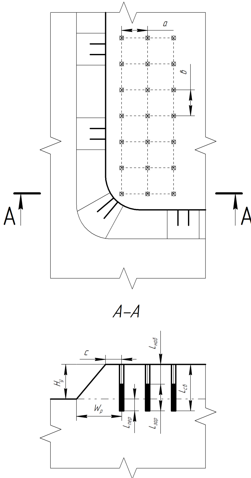
Рис.2.2. Приклад побудови паспорта буровидбухових робіт
