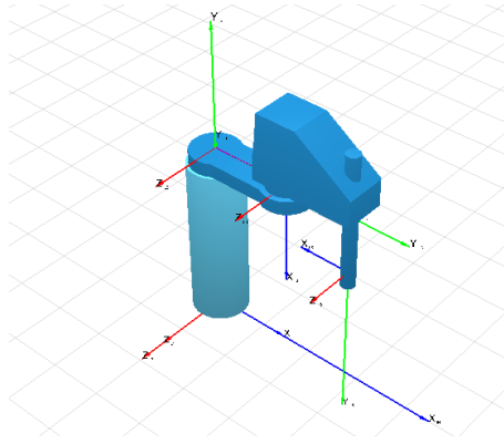
Рис. 5.2.3. Ілюстрація побудованої 3D-моделі МС ПР за ІМ МС ПР
