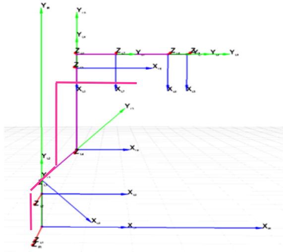
Рис. 5.2.2. Представлення МС ПР мод. KUKA KR-30 у вигляді ниткової моделі (рожевий колір)
