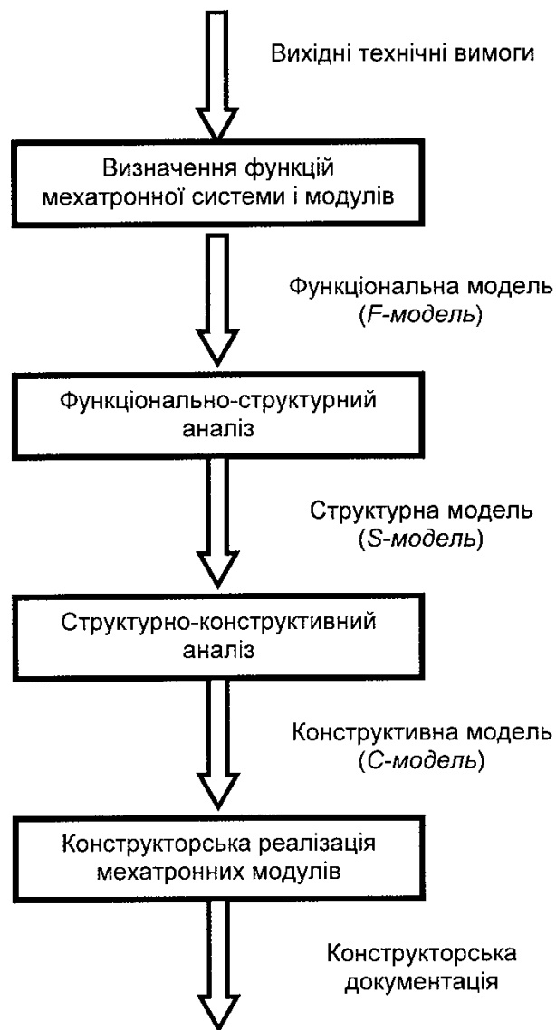
Рис. 6.2 – Загальна процедура проектування МТМ
