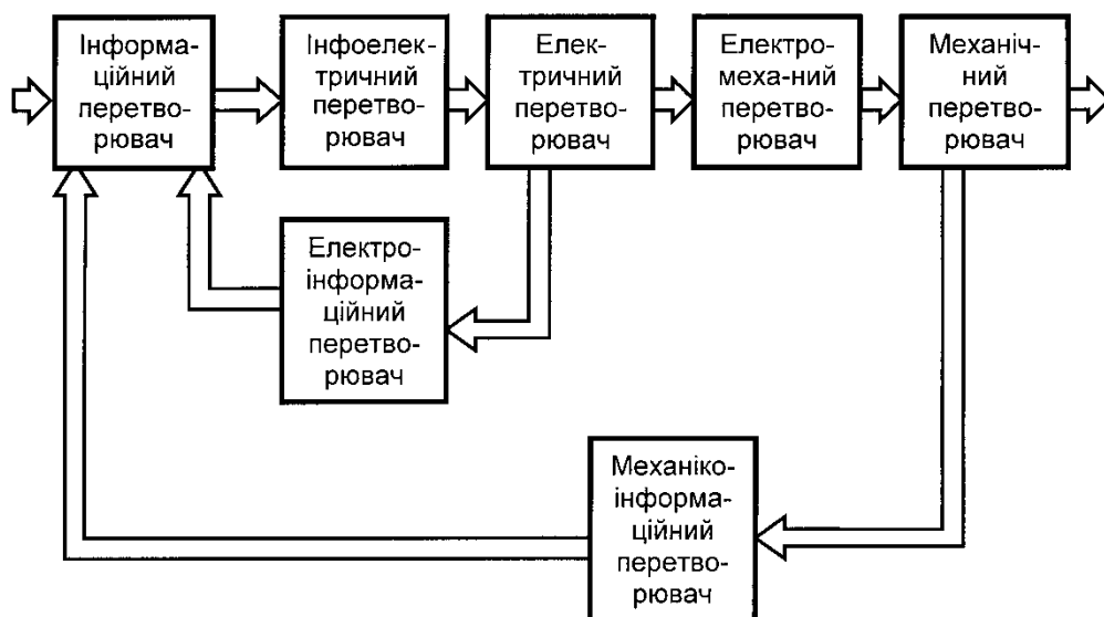
Рис. 6.4. Функціональна модель ( F-модель ) МТМ
