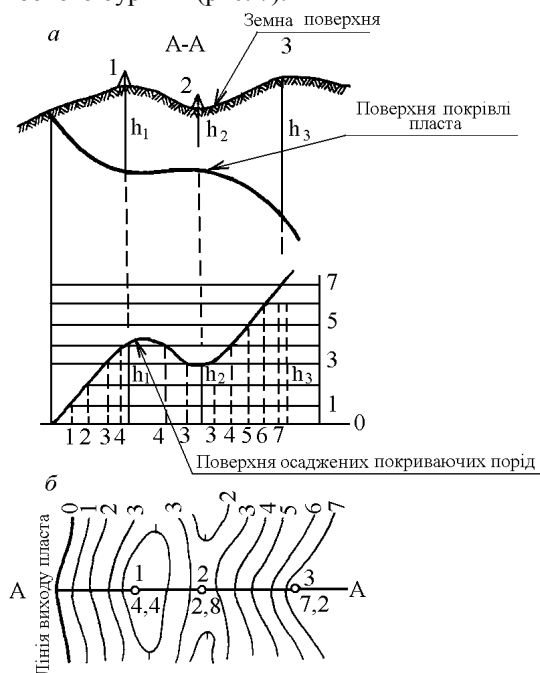
Рис. 7. Побудова ізоглибин залягання пласта (за В. О. Букринським): а – профіль пласта і профіль поверхні;
