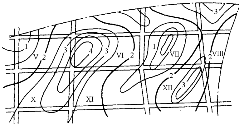
Рис. 17. Ізолінії вмістів корисного компонента ділянки жильного покладу в проекції на похилу площину
