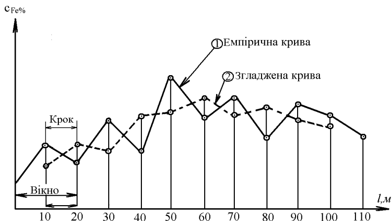
Рис. 15. Згладжування емпіричної кривої методом “ковзного вікна”
