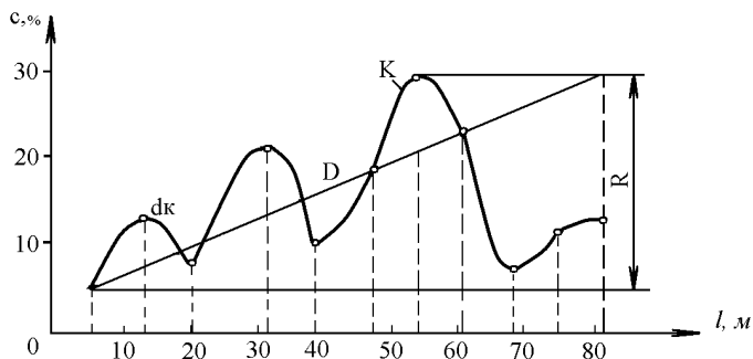
Рис. 22. Графічне зображення реалізації вмісту за В. О. Букринським
