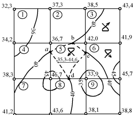
Рис. 25. Побудова плану ізоліній вмісту компонента в руді (за О. Г. Осецьким)
