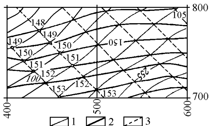
Рис.8. Непрямий спосіб побудови ізоглибин залягання покрівлі: 1 – ізолінії поверхні; 2 – ізогіпси покрівлі пласта; 3 – ізоглибини покрівлі пласта
