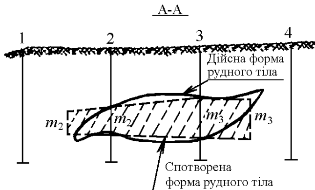
Рис. 1. Спотворення дійсної форми рудного тіла внаслідок лінійного поширення показників
