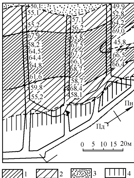
Рис. 13. Частина плану опробування залізорудного покладу: 1 – руда синька; 2 – руда фарбова; 3 – джеспіліти; 4 – фарбові роговики
