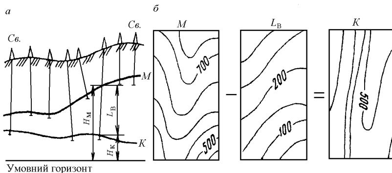
Рис. 5. Схема побудови гіпсометричного плану недостатньо розвіданого пласта K : a – вертикальний розріз; б – віднімання топографічних поверхонь
