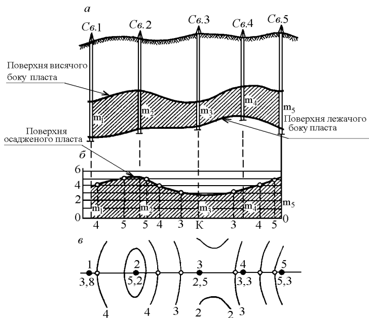
Рис. 6. Побудова ізопотужностей покладу (за В. О. Букринським):
