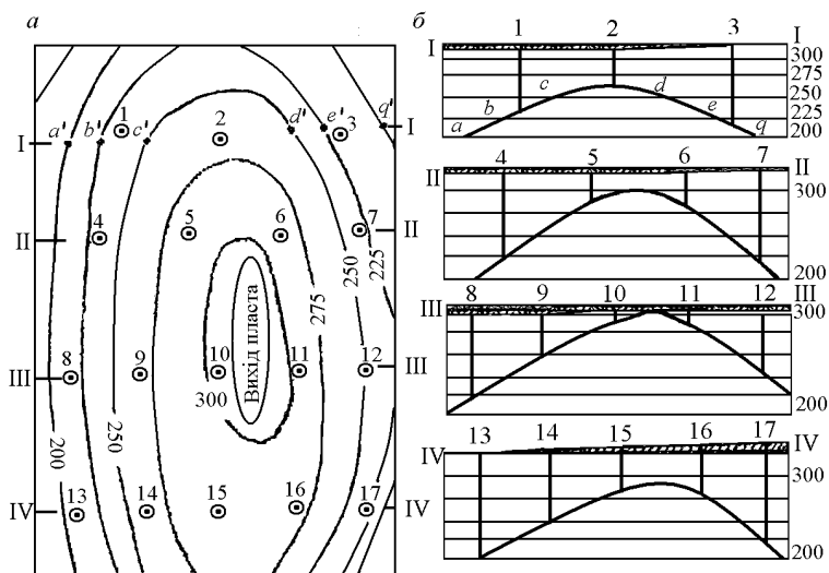
Рис. 4. Побудова гіпсометричного плану (а) за вертикальними розрізами (б)
