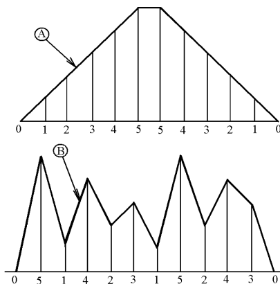
Рис. 20. Два розрізи з однаковими статистичними характеристиками, але з різною величиною мінливості
