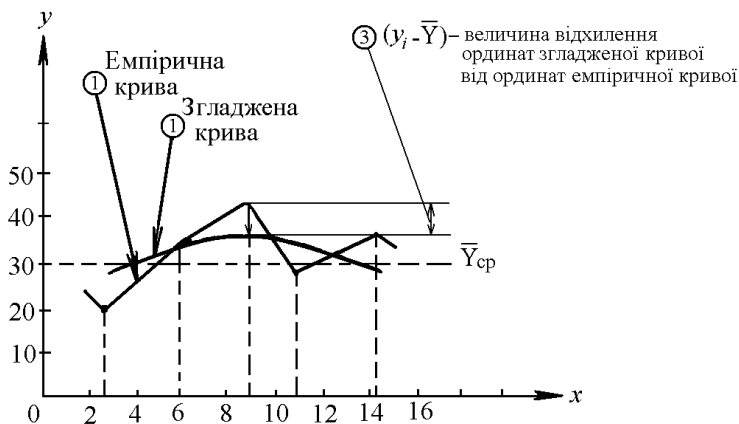
Рис. 18. Побудова кривої регресії
