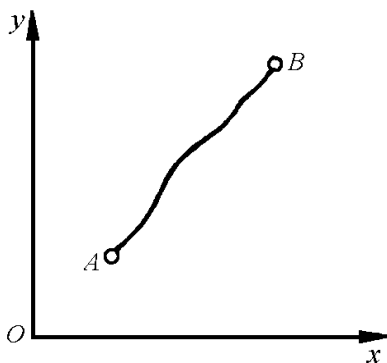
Рис. 2. Графічне зображення функції однієї змінної
