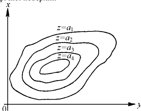
Рис. 3. Графічне зображення функції двох змінних
