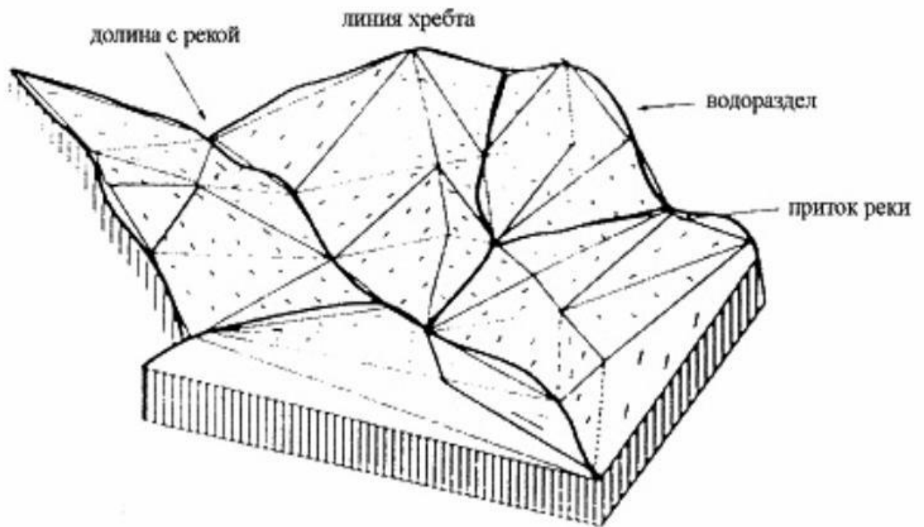
Рис. 1. TIN модель
