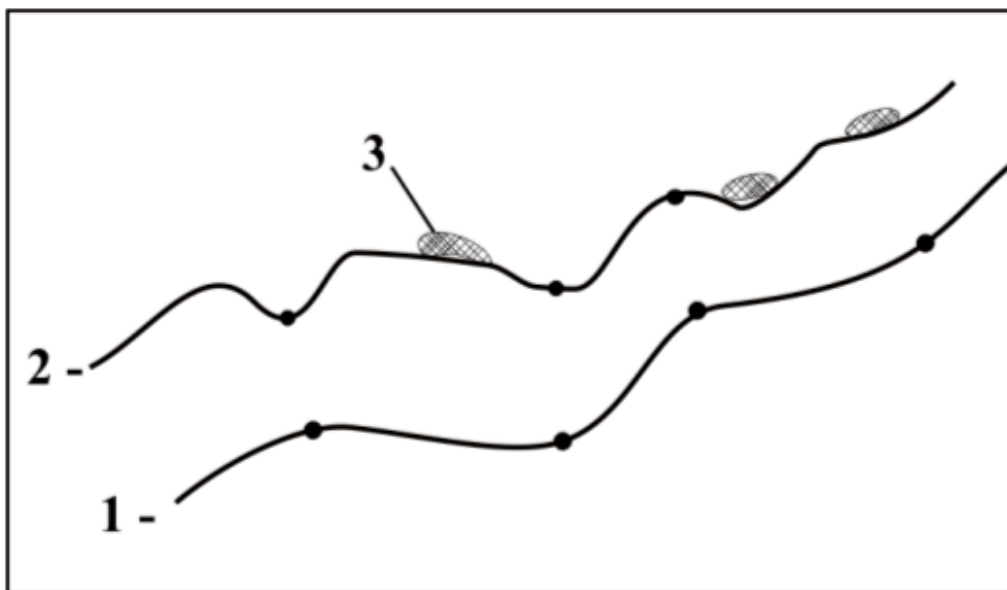
Рис. 4. Елементи кригинга :
