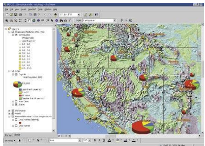
Рис. 3. ГІС-застосунки
