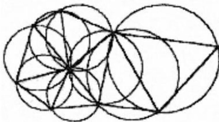
Рис. 2. Триангуляція Делоне
