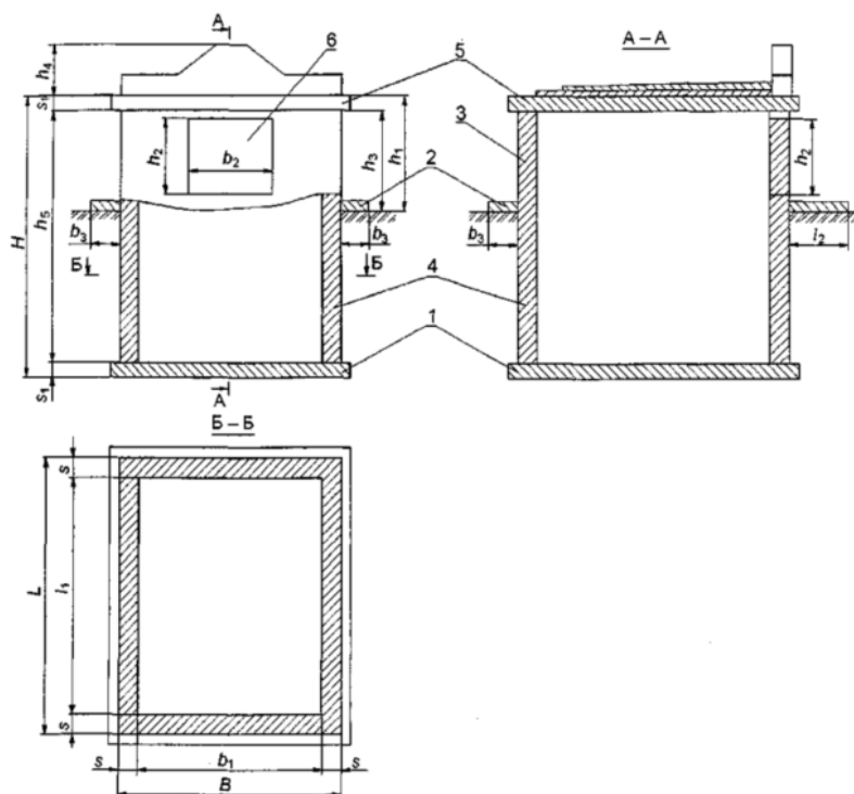
Рис.30. Типовий склеп та його складові елементи з боковим розміщенням входу для занесення померлого: 1 – наземна частина; 2 – вхід; 3 – відмостка; 4 – підземна частина; 5 – елементи благоустрою
