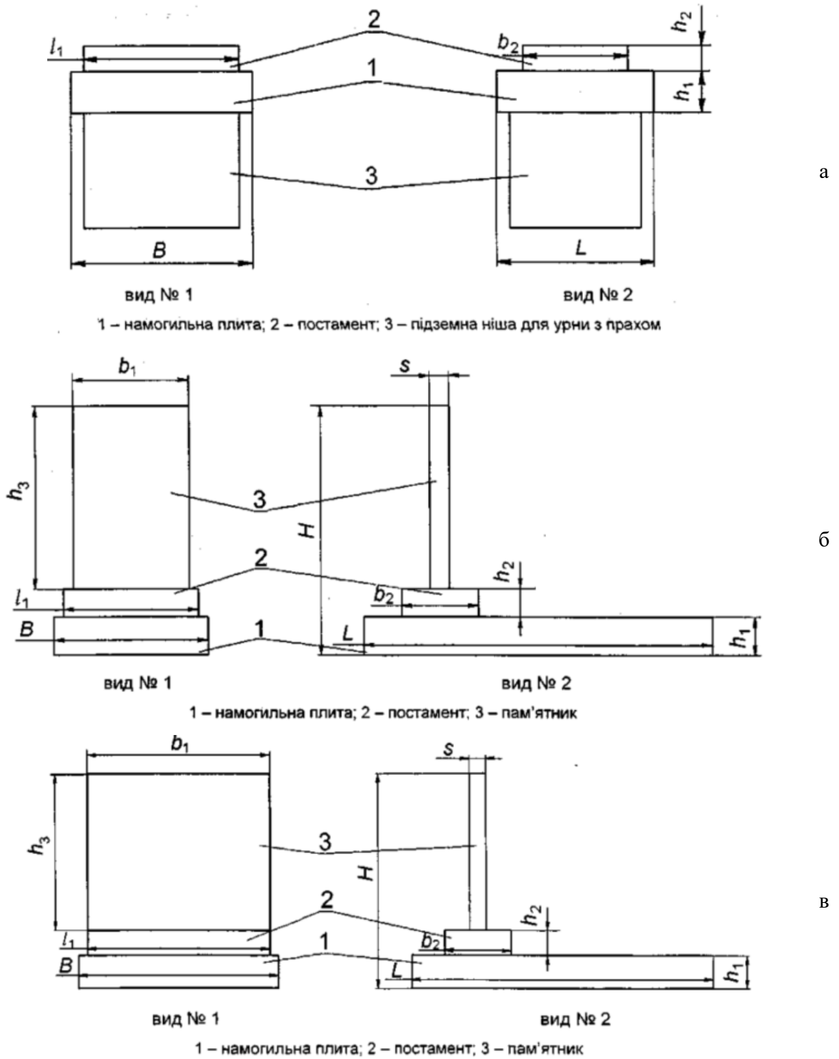
Рис.29. Основні конструкції намогильних споруд: а – намогильна споруда на місці поховання урн з прахом; б – намогильна споруда на місці одинарного поховання; в – намогильна споруда на місці подвійного чи родинного поховання.
