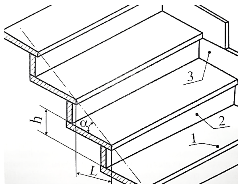
Рис.16. Конструкція сходів з покритими сходинокми: 1 – сходинок; 2 – підсходинок; 3 – плінтус.
