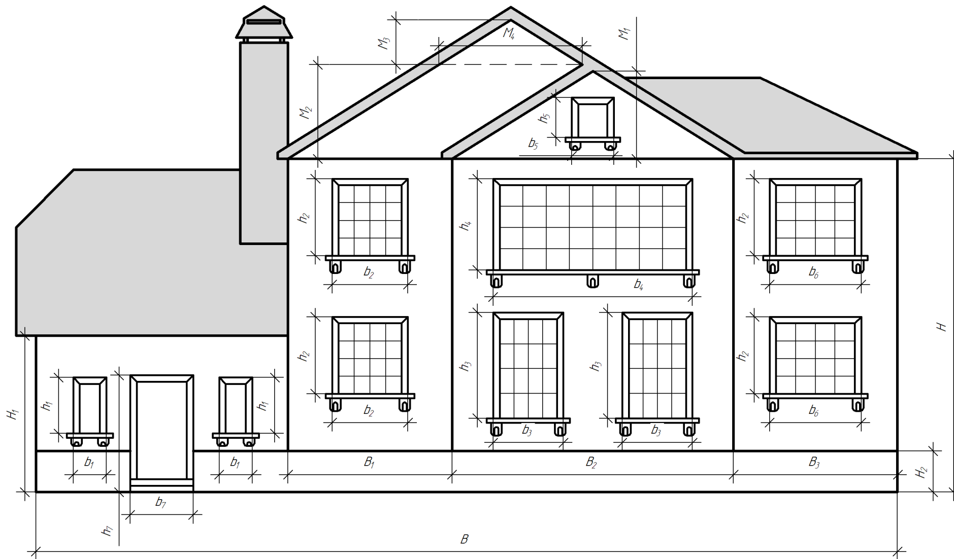
Рис. 17. Схема лицьової сторони фасаду будинку
