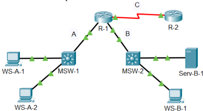
Рис.9. Приклад мережі
