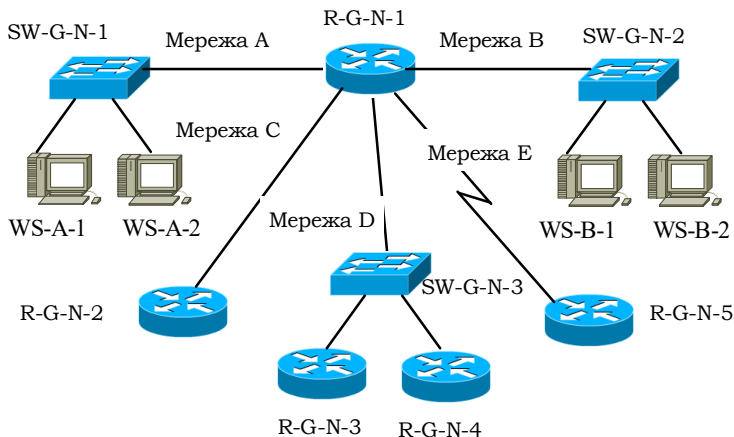
Рис. 19 Проєкт мережі
