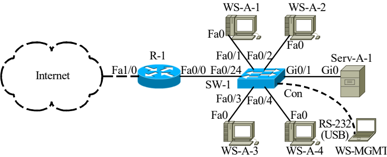
Рис. 17. Приклад мережі
