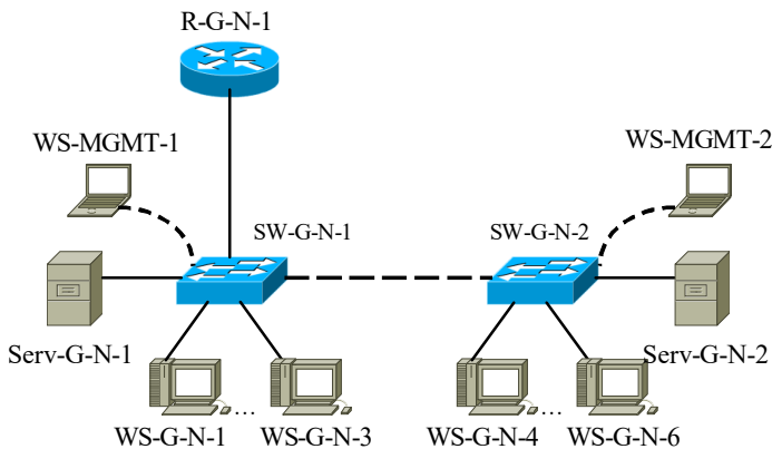
Рис. 28. Проєкт мережі
