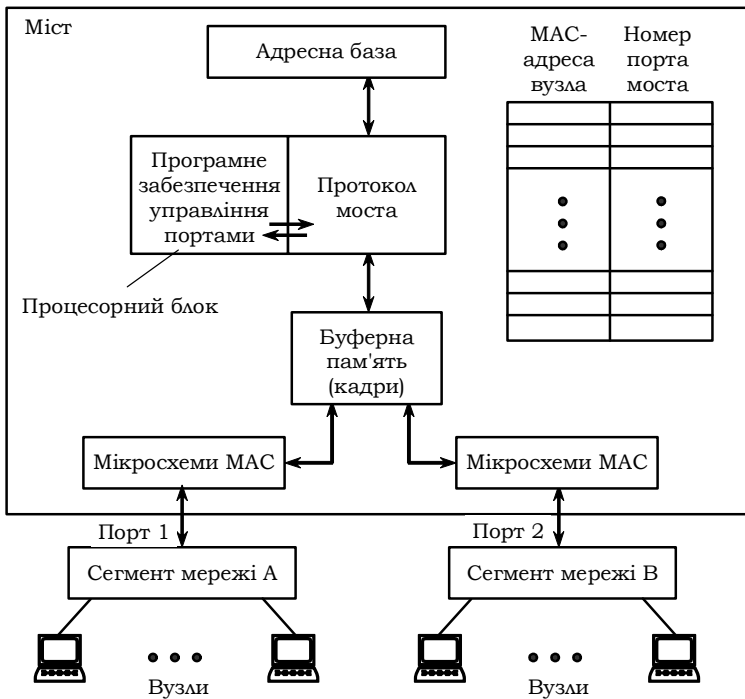
Рис. 1. Структура моста
