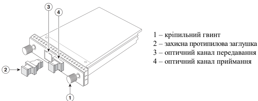
Рис. 7. Мережний інтерфейсний модуль CFP
