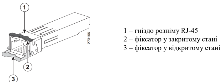
Рис. 4. Мережний інтерфейсний модуль SFP (рознім RJ-45)
