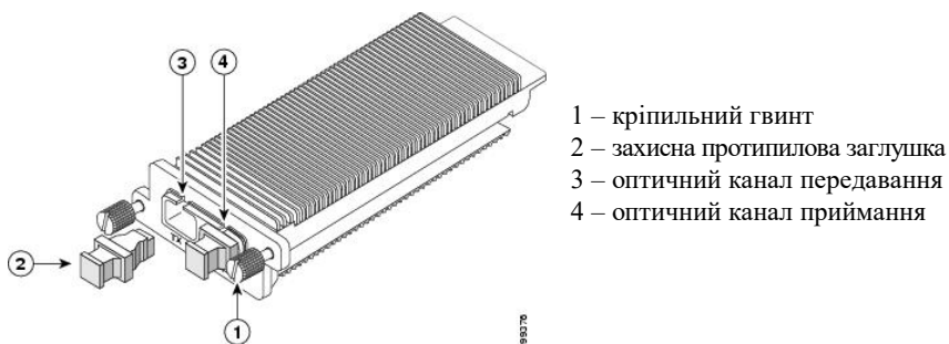
Рис. 8. Мережний інтерфейсний модуль XENPAK
