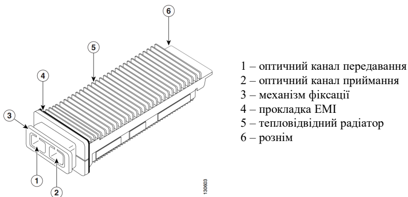
Рис. 9. Мережний інтерфейсний модуль X2
