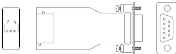
Рис. 8. RJ-45–DB-9 Adapter
