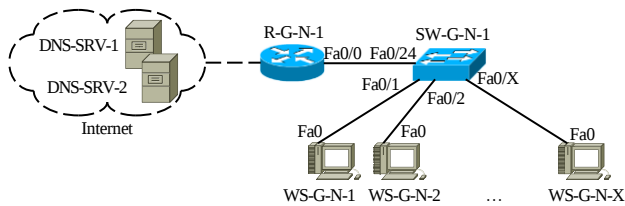
Рис. 14. Проект мережі
